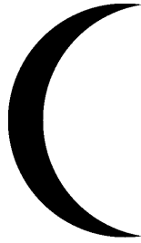
Figura 3.4. Desenho da diferença de duas regiões circulares
